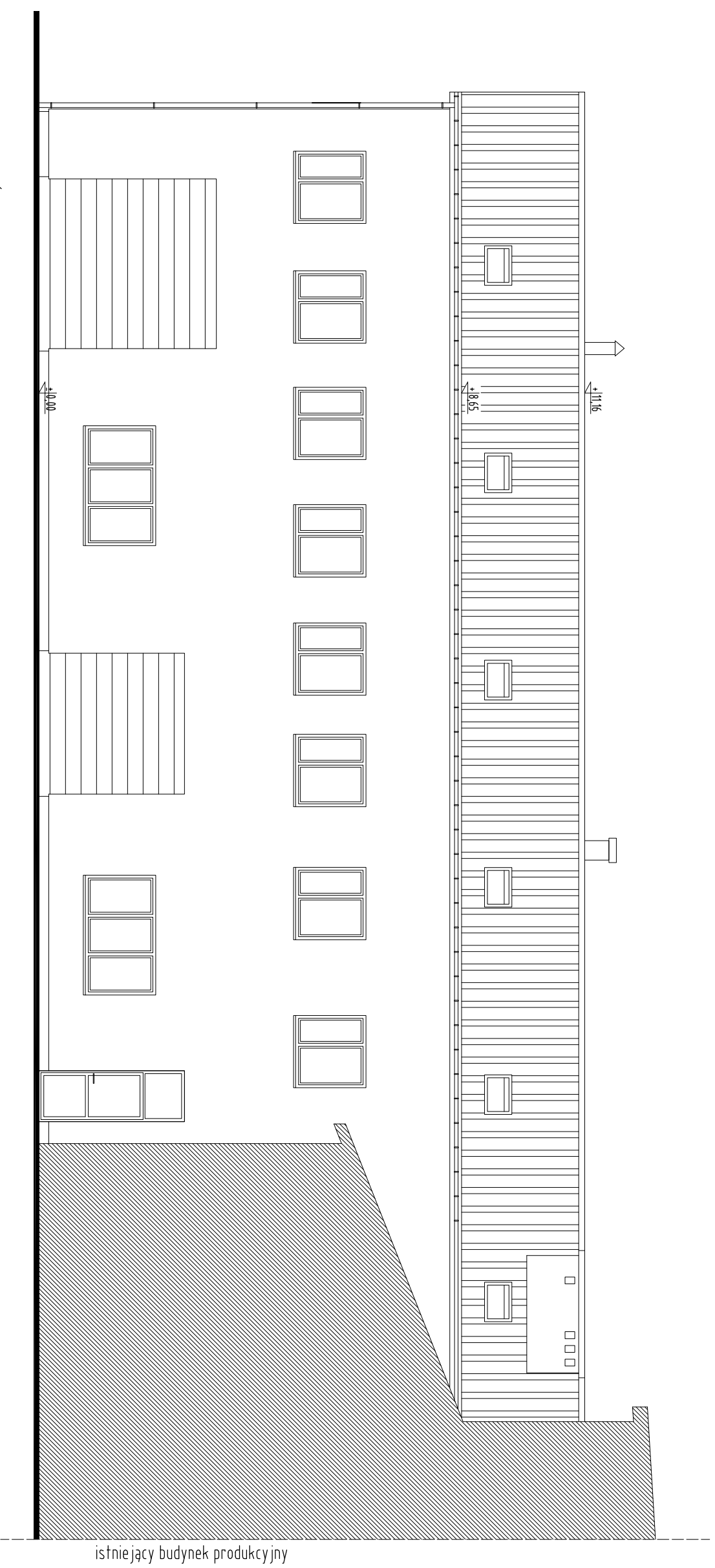
ELEWACJA PÓŁNOCNA - STAN PROJEKTOWANY
